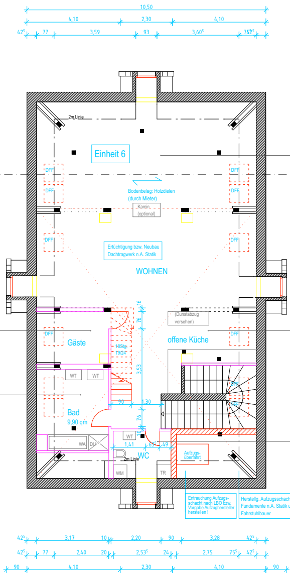
GRUNDRISS DACHGESCHOSS
