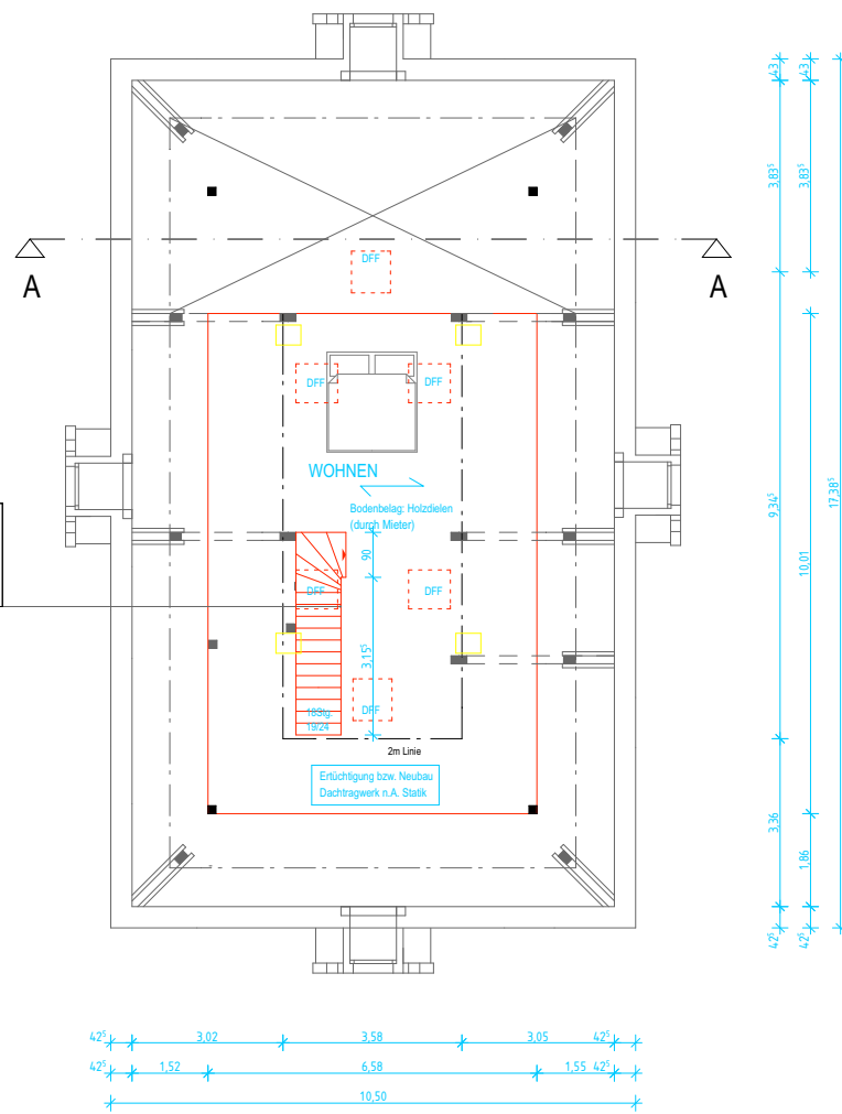
GRUNDRISS GALERIE
